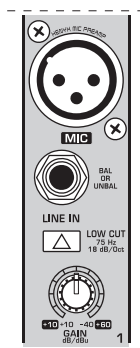
Рис. 2.1: Соединительные элементы и регулятор Mic-/Line-входов
