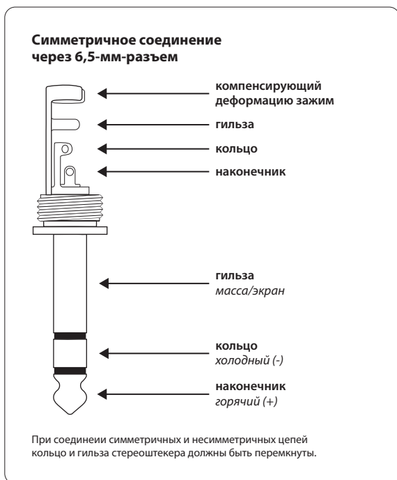
Рис. 3.3: 6,3-мм-стереохраповый штекер
