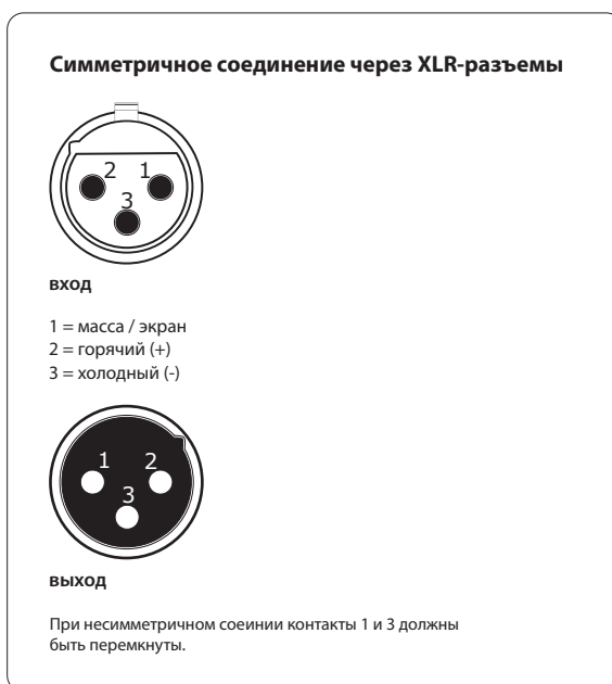
Рис. 3.1: XLR-соединения
