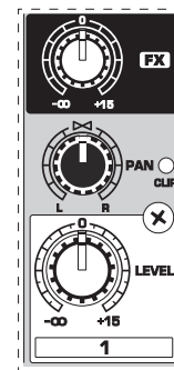
Рис. 2.3: FX Send/Panorama/Level-регулятор
