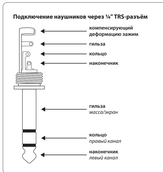
Рис. 3.4: Стереохраповый штекер для наушников
