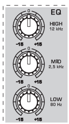
Рис. 2.5: Настройка звучания каналов со стереовходами
