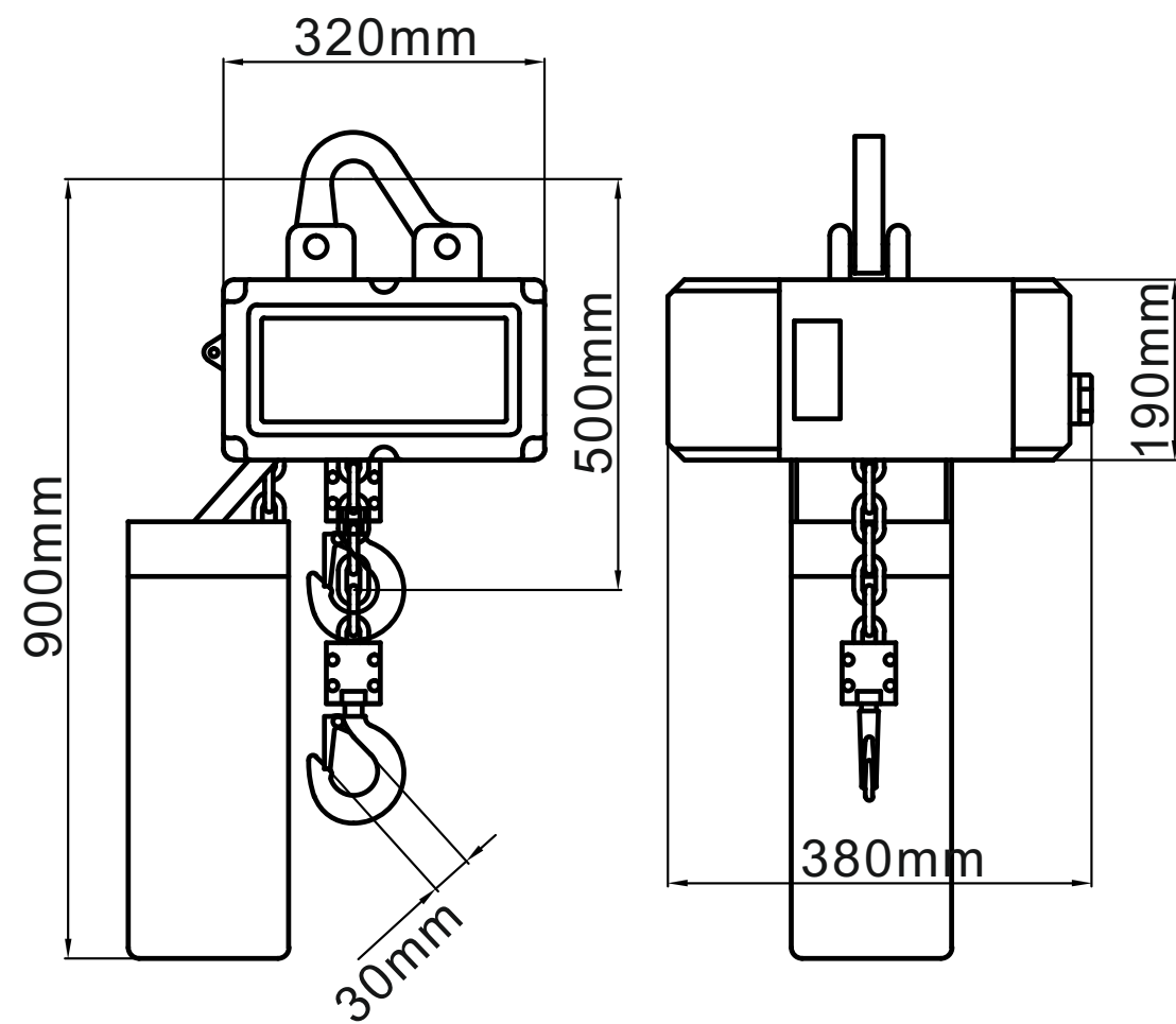
Размеры ST-1000
