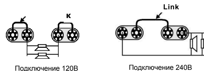
Рис 3. Соединения
