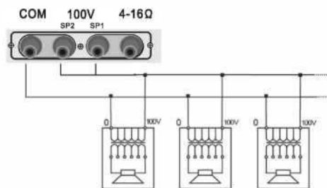
Подключение нескольких динамиков параллельно к выходу 100 В
