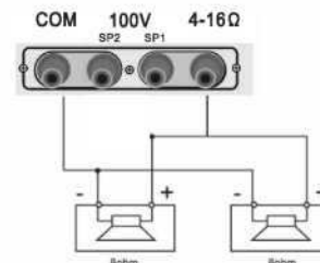
Подключение двух громкоговорителей по 8 Ом к выходу 4 Ом параллельно
